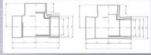
Tee, T-Stück, Te
